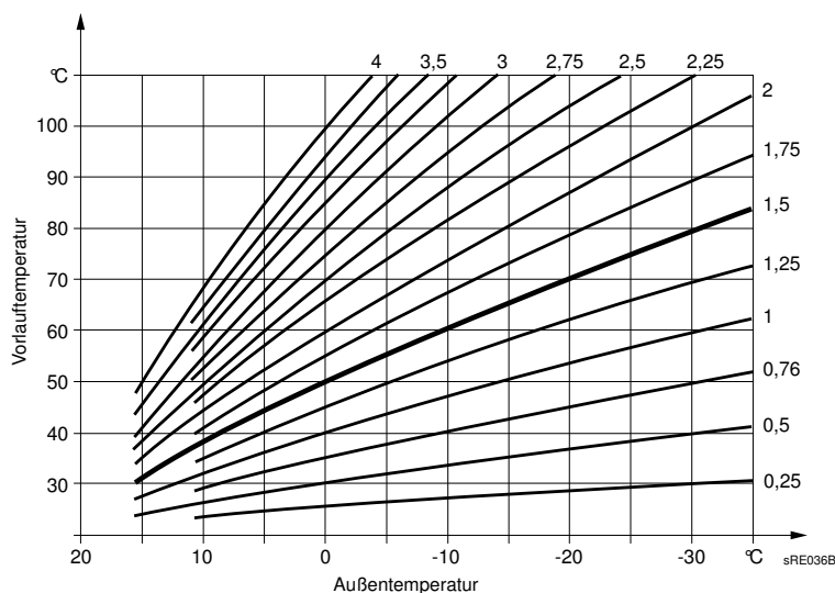
Abb. 4: Heizkennlinie
